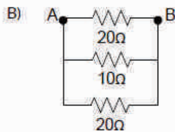
Figura. Exemplo de Associação de Resistores em Paralelo
