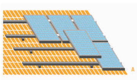
Figura: Instalação na extremidade
